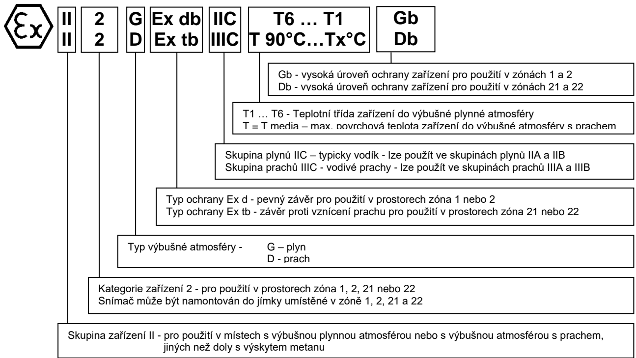
OBRÁZEK 5 - OZNAČENÍ NEVÝBUŠNOSTI
