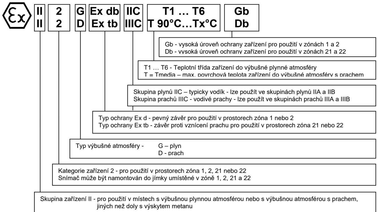
OBRÁZEK 3 - OZNAČENÍ NEVÝBUŠNOSTI
