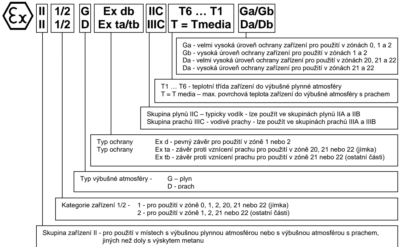
OBRÁZEK 4 - OZNAČENÍ NEVÝBUŠNOSTI
