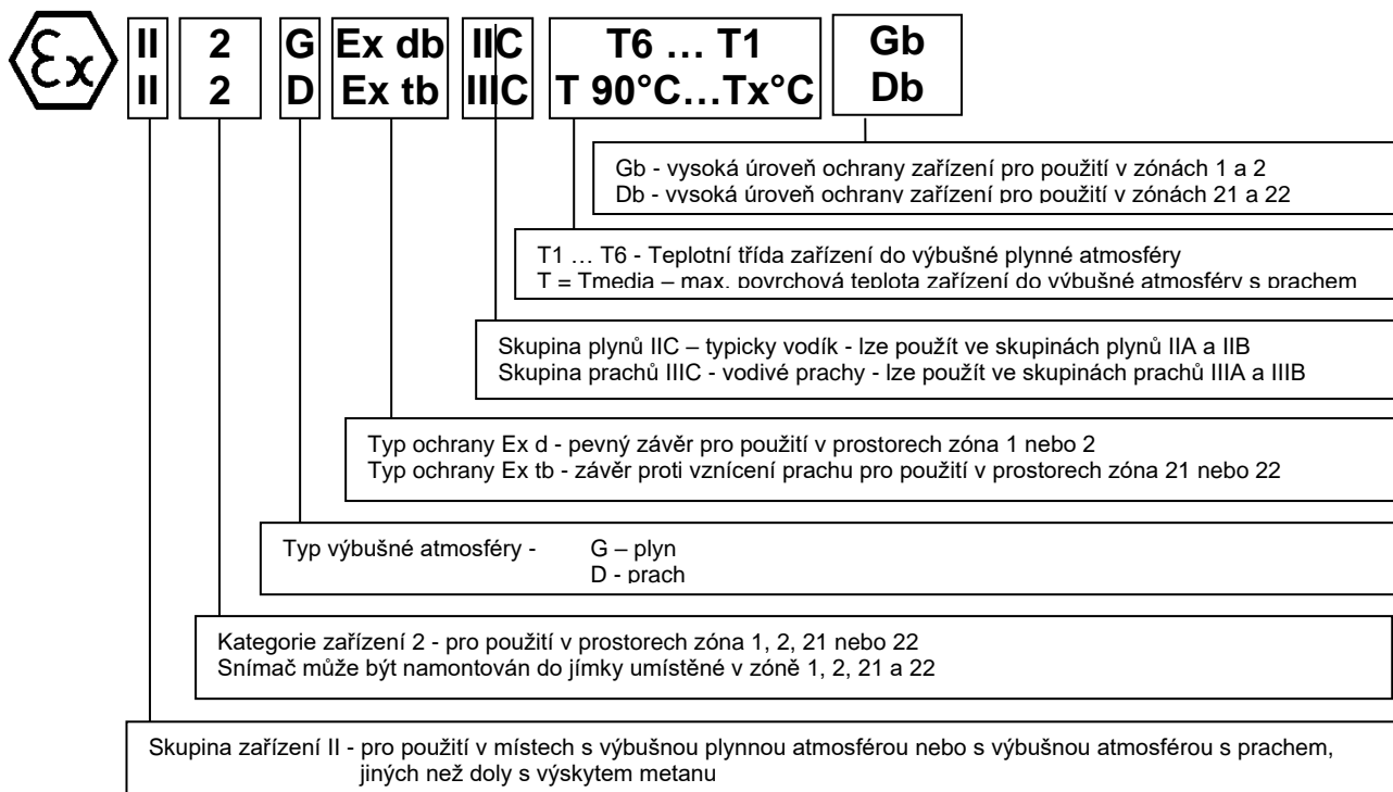
OBRÁZEK 6 - OZNAČENÍ NEVÝBUŠNOSTI
