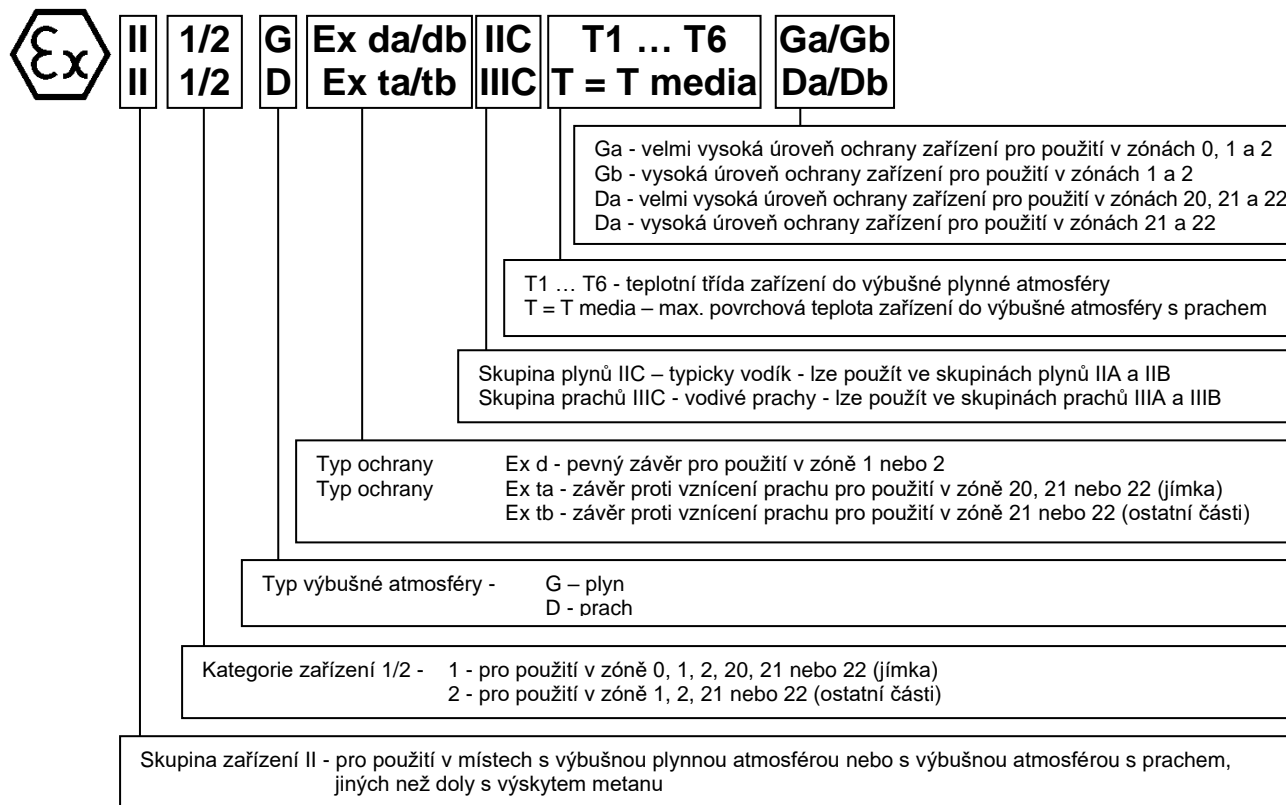
OBRÁZEK 5 - OZNAČENÍ NEVÝBUŠNOSTI
