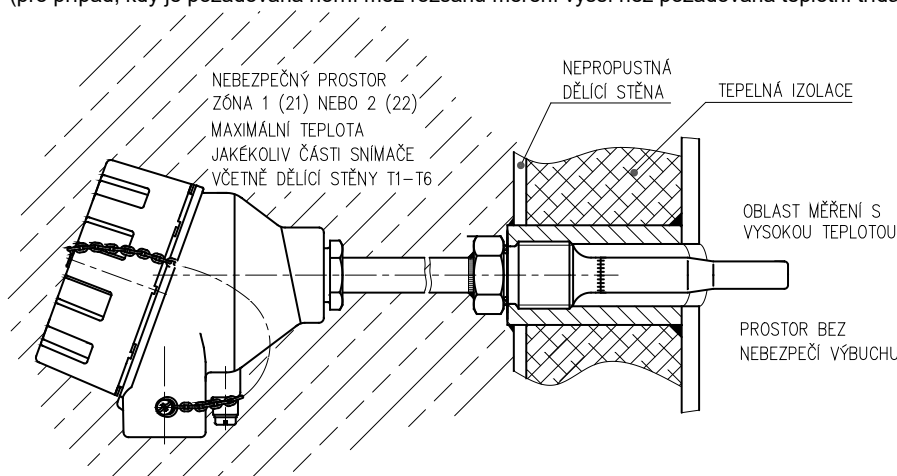
OBRÁZEK 6 - OZNAČENÍ NEVÝBUŠNOSTI
