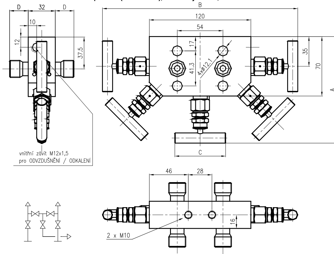
Obrázek 17 - Pěticečná ventilová souprava (964 45.. AS2), rozměrový nákres, schéma
