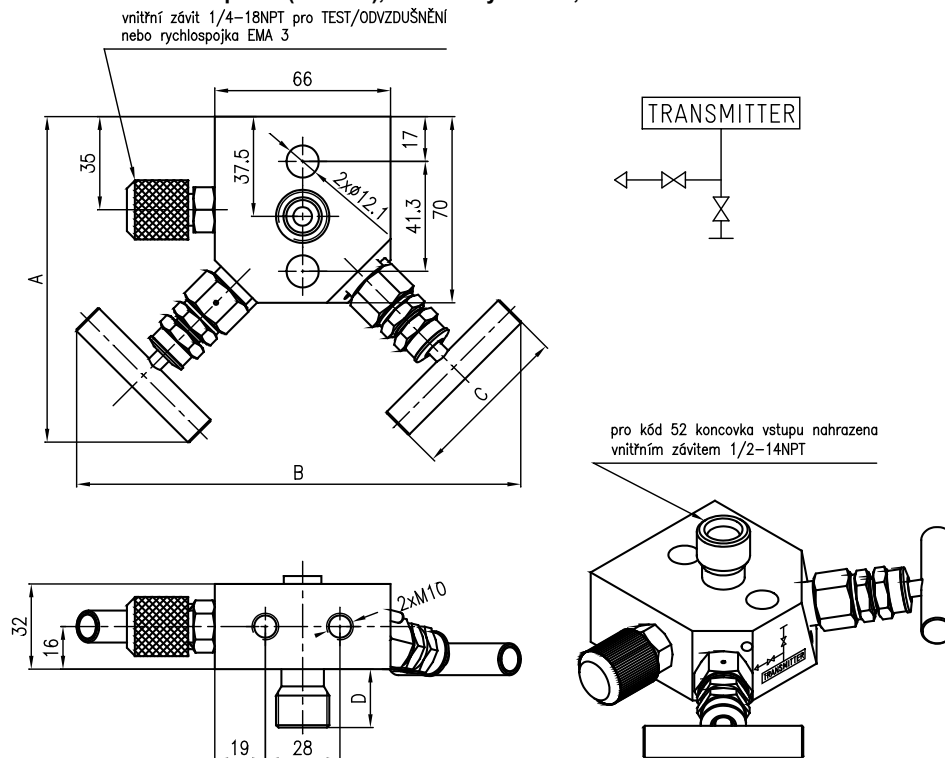
Obrázek 2 - Dvoucestná ventilová souprava (964 21..), rozměrový náčrtek, schéma
