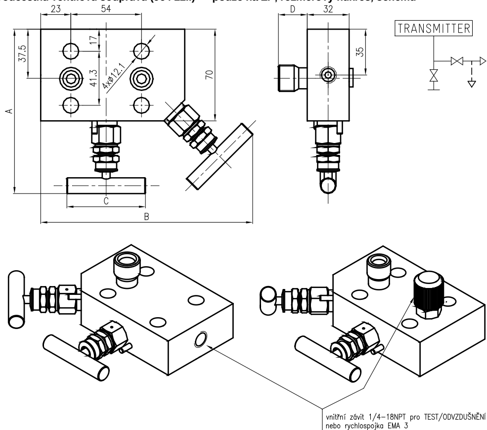
Obrázek 3 - Dvoucestná ventilová souprava (964 22..) pouze na ZP, rozměrový náčrtek, schéma
