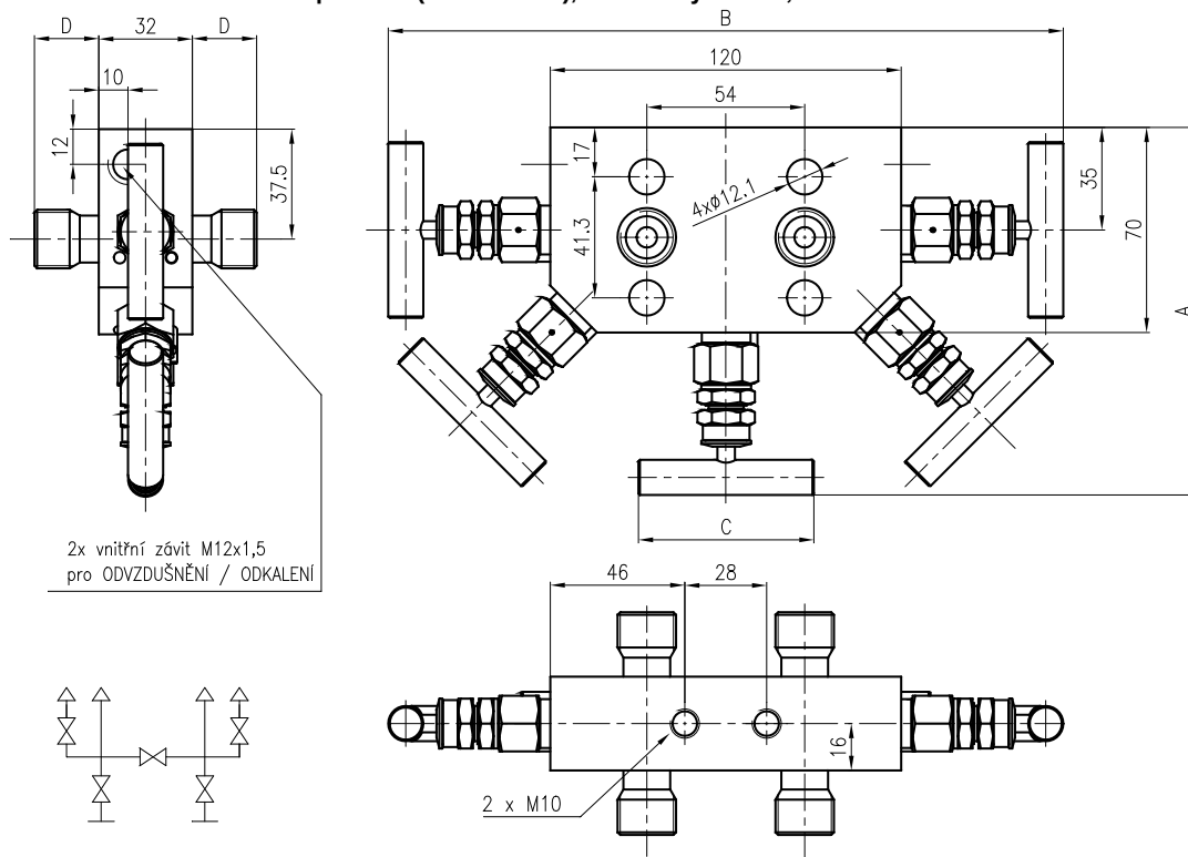
Obrázek 16 - Pěticečná ventilová souprava (964 45.. AS1), rozměrový nákres, schéma
